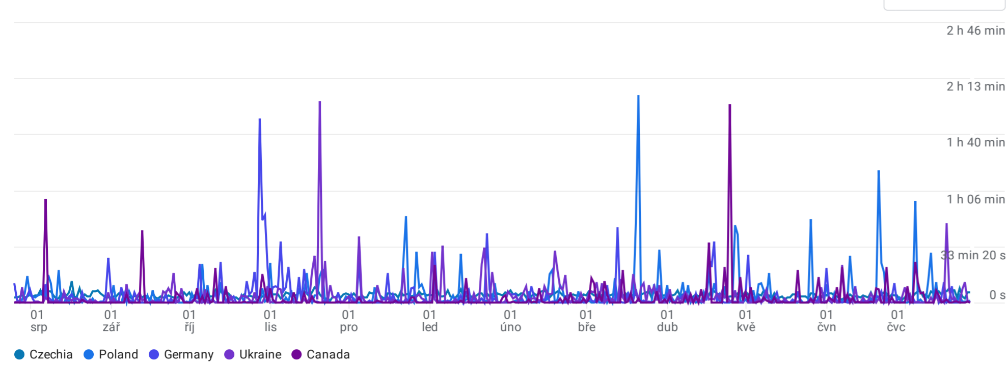
Průměrná doba zapojení podle Země v průběhu času
